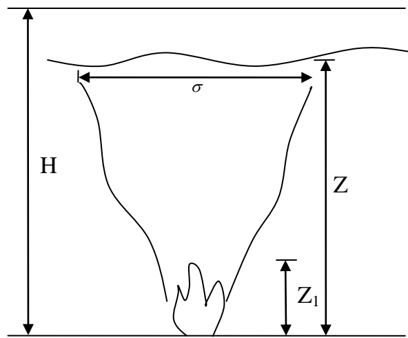
图 10 轴对称型烟缕
