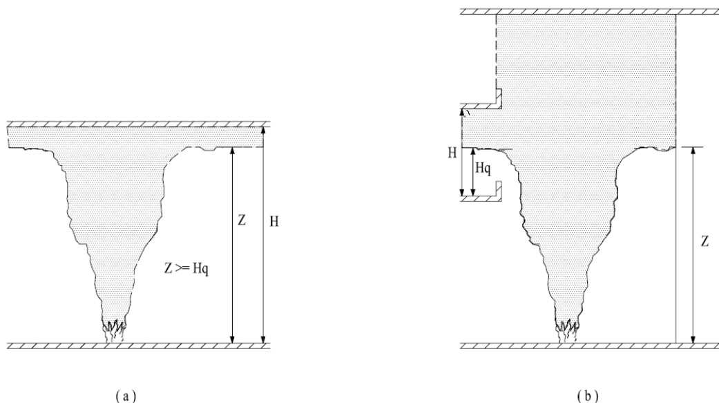
图9 最小清晰高度示意图
