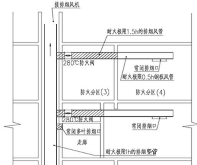
图 7 排烟管道布置示意图
