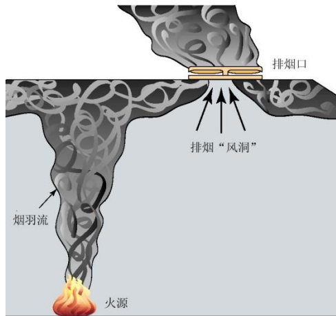
图 15 排烟口的最高临界排烟量示意图
