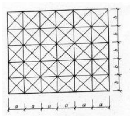
图 17 矩形风管测点布置图
