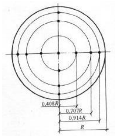
图 18 圆形风管测点布置图
