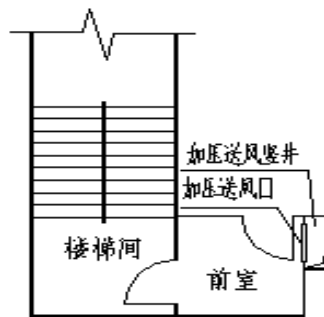
图 1 挡住加压送风口的疏散门
