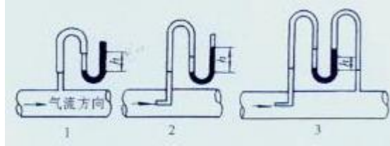
图 19 用 U 形管压力计测定风压
