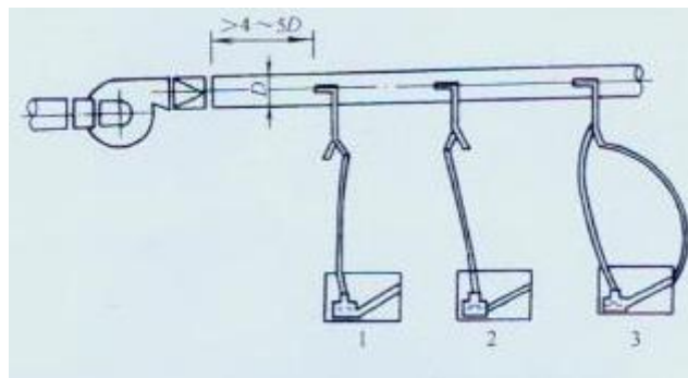
图 21 压出段毕托管与倾斜式微压计的联接方法
