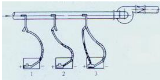
图 20 吸入段毕托管与倾斜式微压计的联接方法
