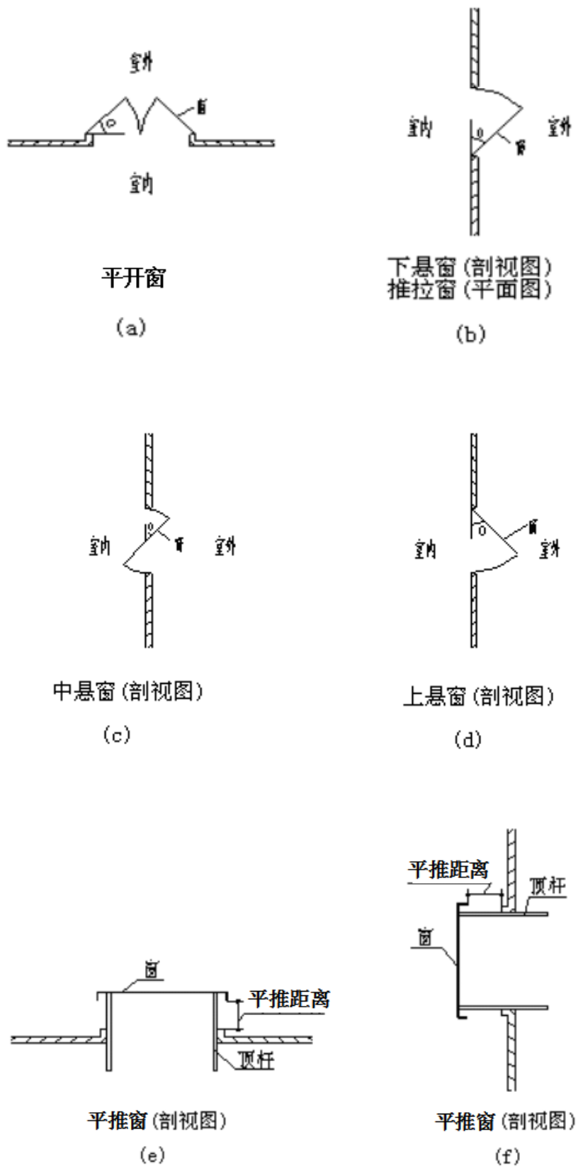
图 6 可开启外窗的示意图
