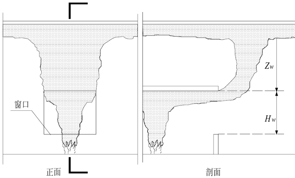
图 12 窗口溢出型烟缕
