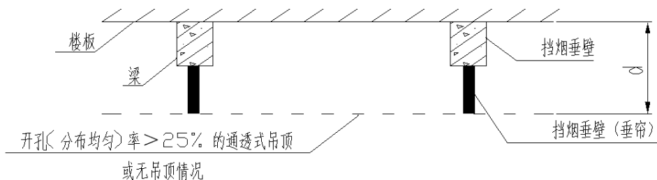
图 3 无吊顶或设置开孔（均匀分布）率>25%的通透式吊顶
