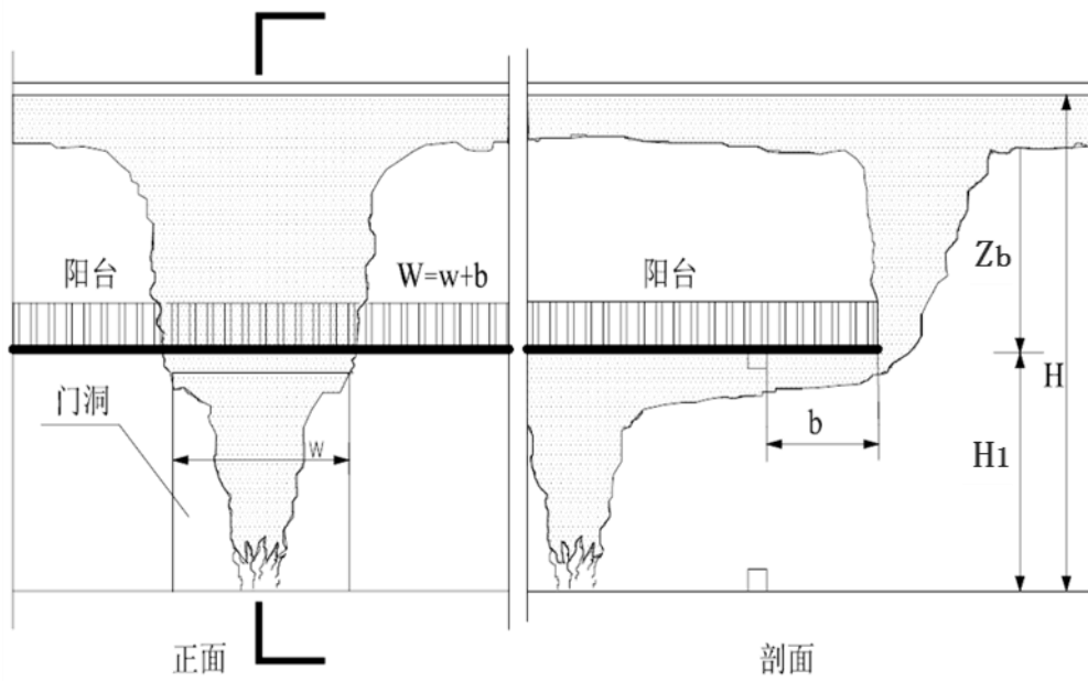
图 11 阳台溢出型烟缕
