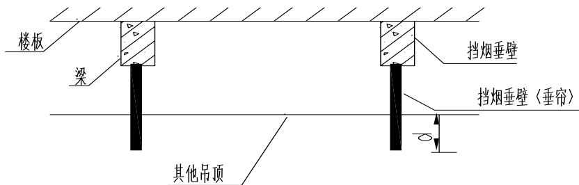
图 4 开孔率 \leq 25\% 或开孔不均匀的通透式吊顶及一般吊顶
